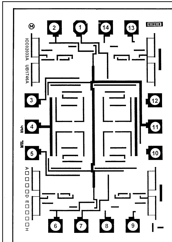
MPC102AD DIE TOPOGRAPHY
